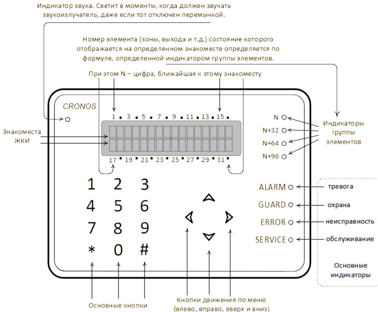
Рисунок 1.1 Внешний вид клавиатуры (передняя панель, вид спереди)
