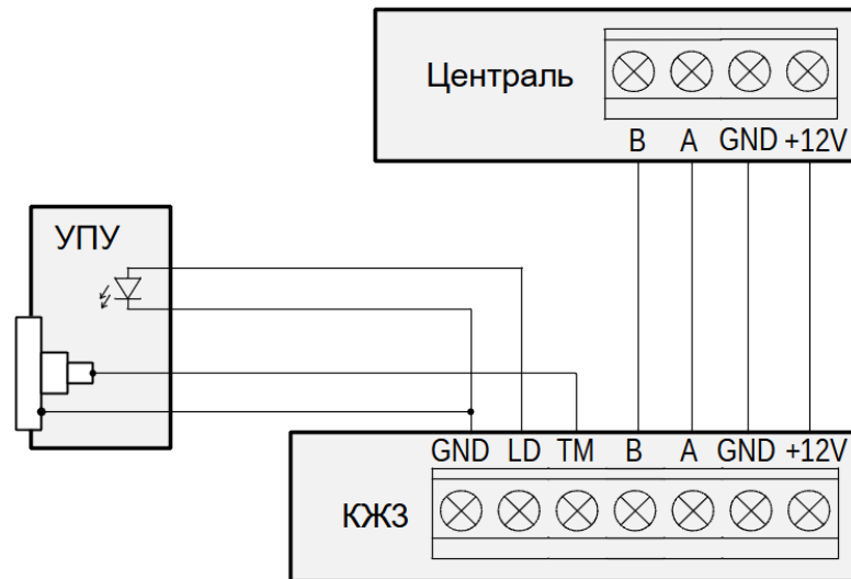
Рисунок 5.2 Схема подключения.
