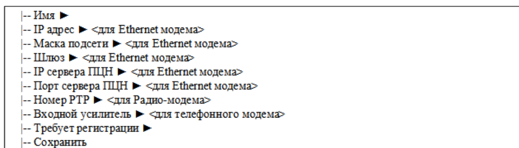
Рисунок 4.49. Структура подменю параметров модема.
