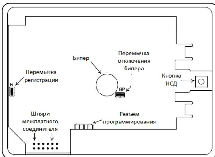
Рисунок 3.1 Разъемы и перемычки, расположенные на передней панели клавиатуры (вид на переднюю панель сзади, после отделения ее от задней панели).
