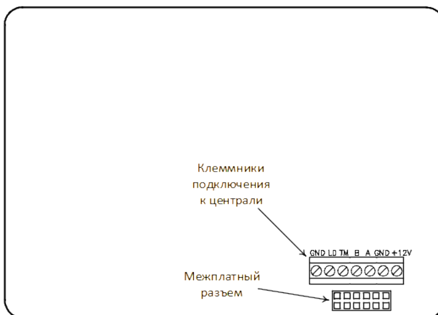
Рисунок 3.2 Клеммники и разъем, расположенные на задней панели клавиатуры (вид после отделения от передней панели).
