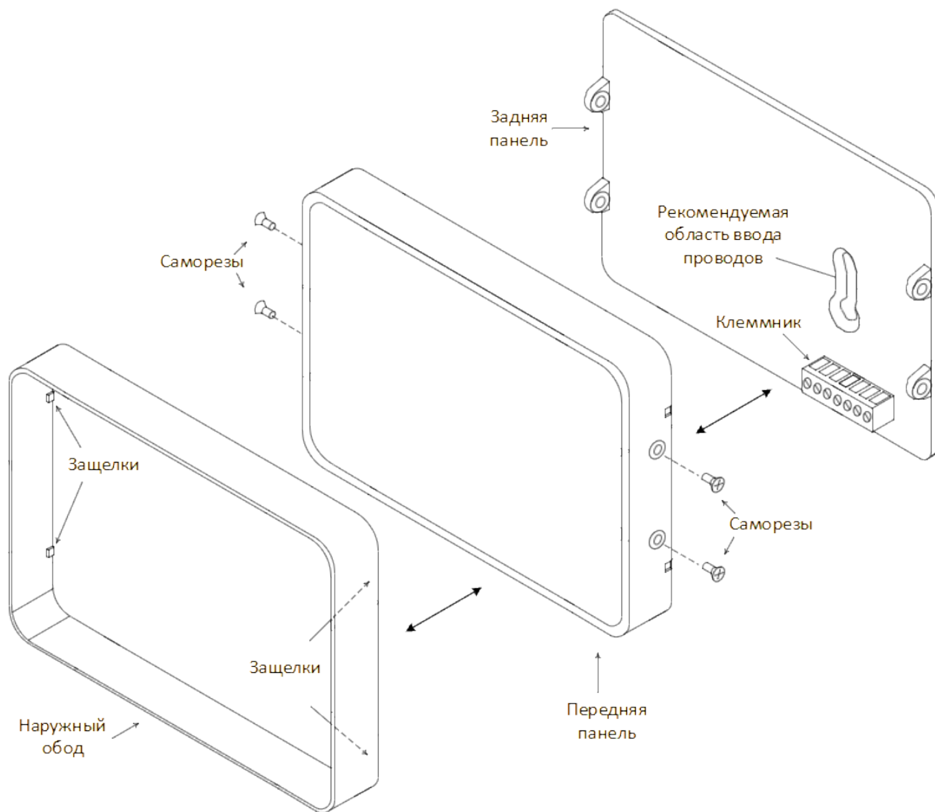
Рисунок 5.1 Составные элементы клавиатуры.
